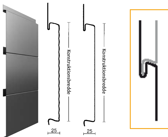
Uden skyggefuge Skrå fuge Med / uden mikroliniering Opsætning nede fra og opad
