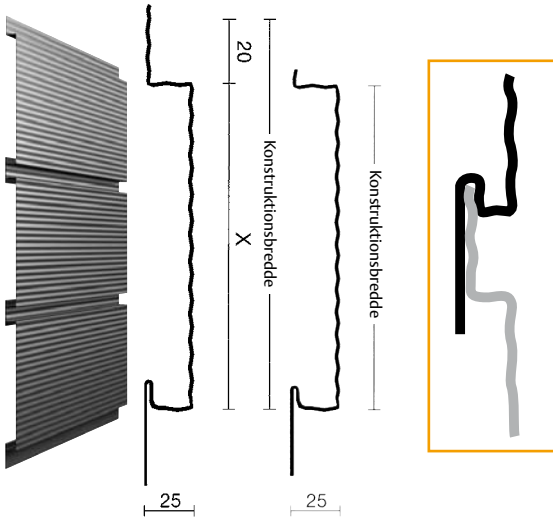
Med / uden skyggefuge (20 mm) Lige Fuge Med mikroliniering Opsætning oppe fra og nedad
