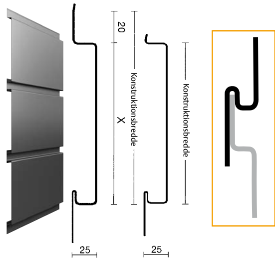
Med / uden skyggefuge (20 mm) Lige Fuge Uden mikroliniering Opsætning oppe fra og nedad
