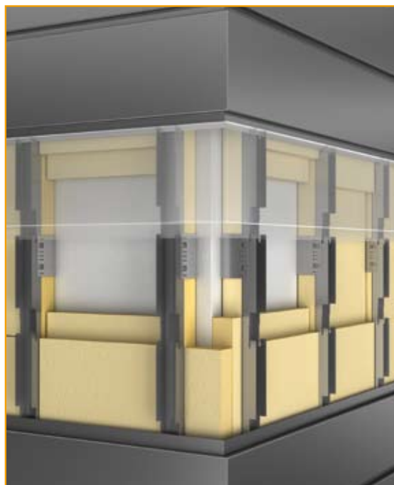
Underkonstruktion med modulliste
